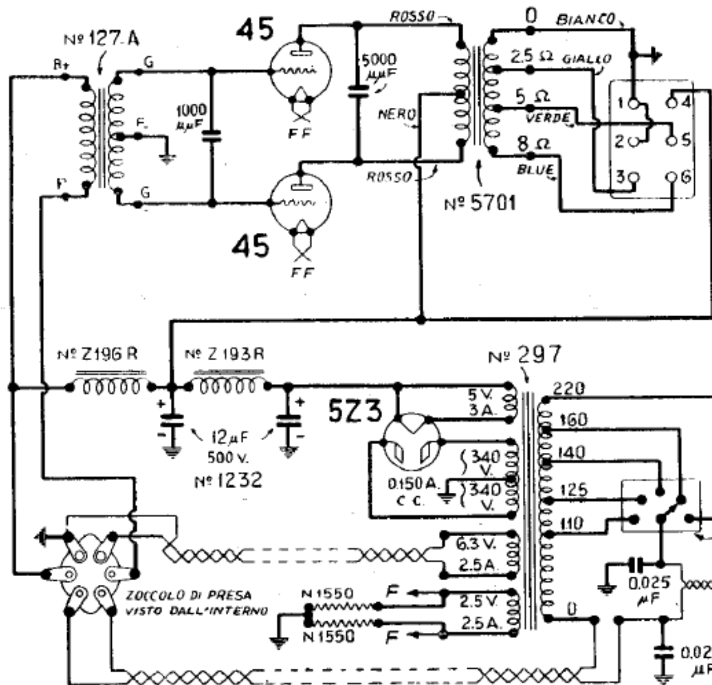
Schema elettrico (Chassis alimentazione e B.F.).
